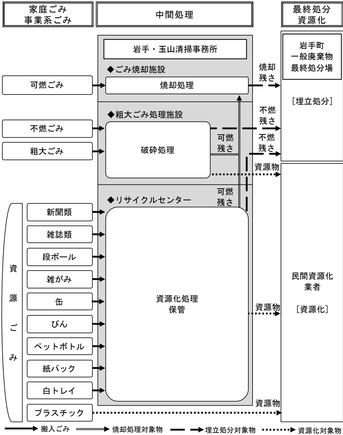
図 3-2 ごみ処理体系 (岩手町)
