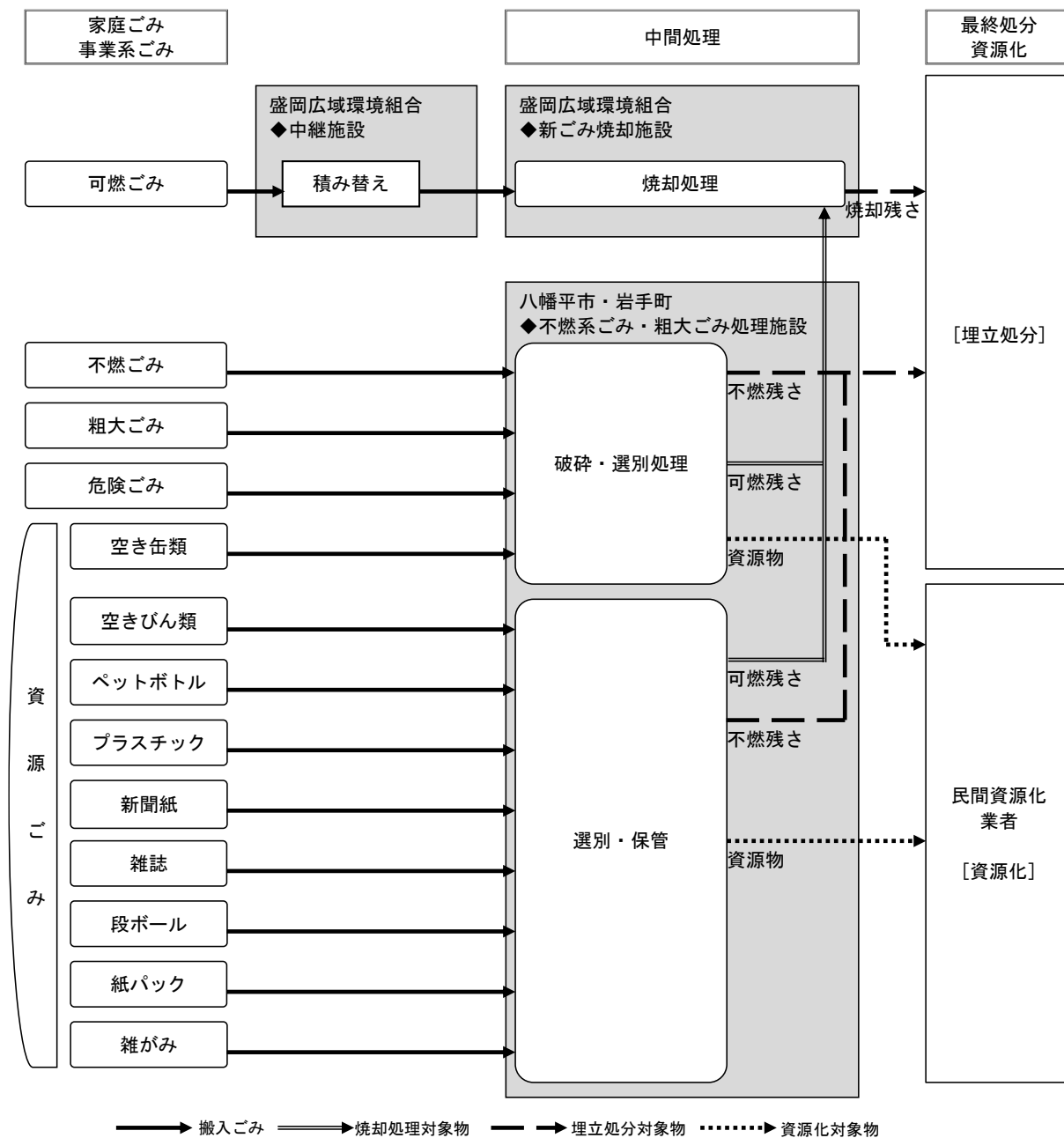
図 5-5 中継施設稼働後のごみ処理体系（八幡平市）
