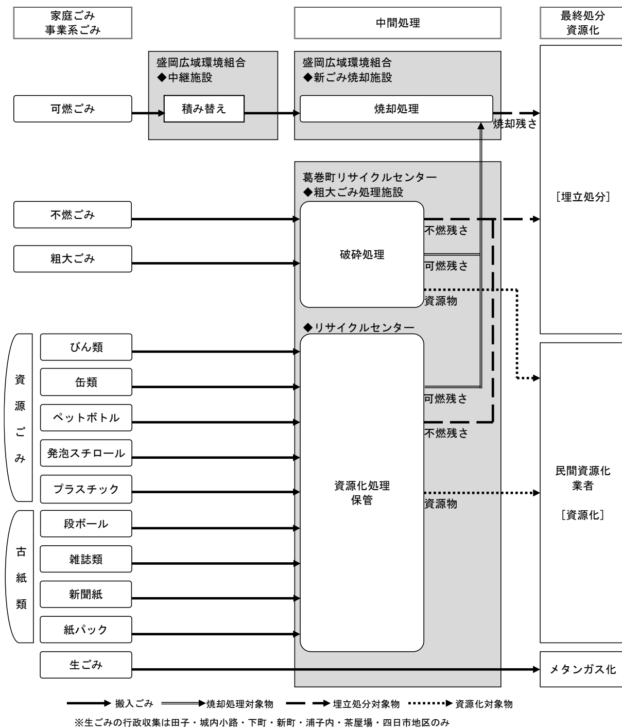
図 5-7 中継施設稼働後のごみ処理体系 (葛巻町)
