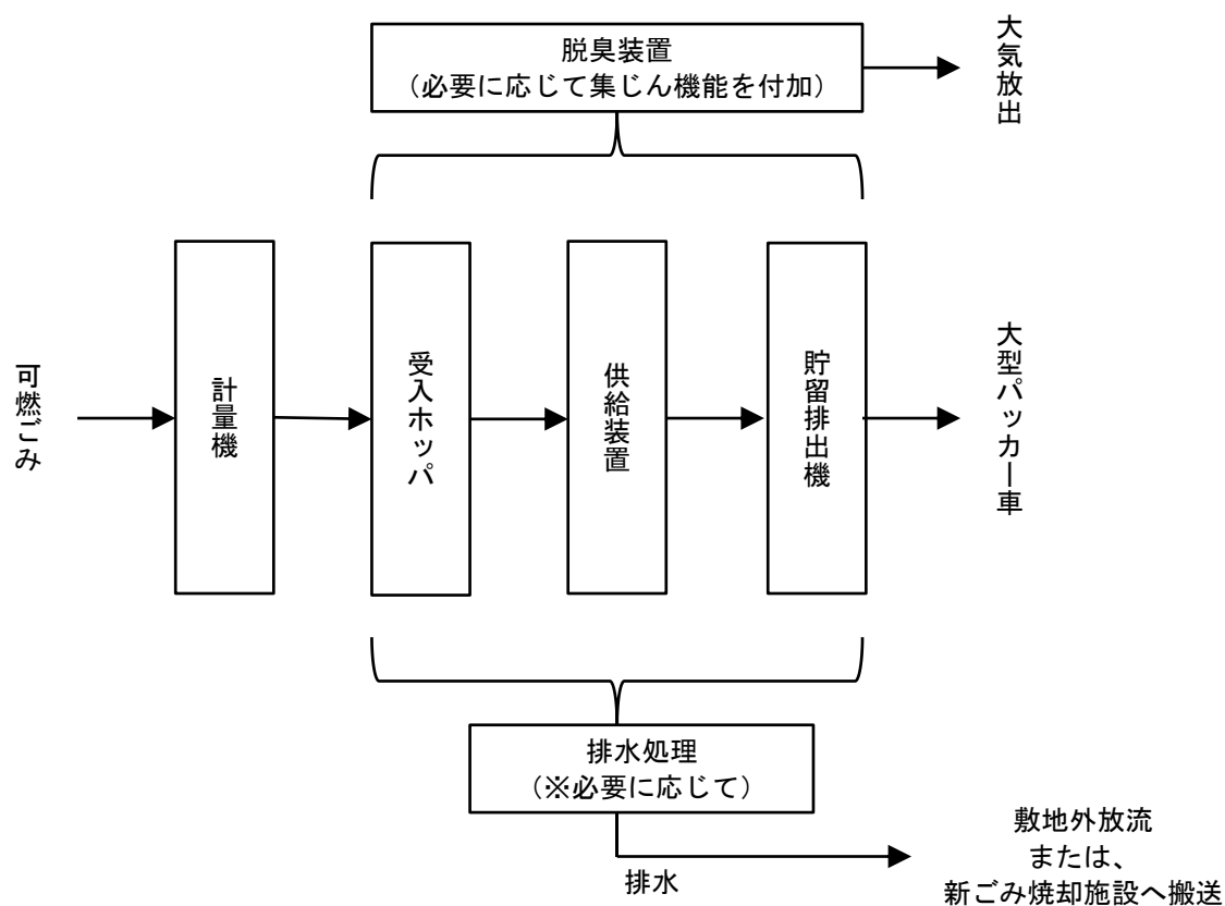
図 8-2 貯留排出機方式の基本処理フロー
