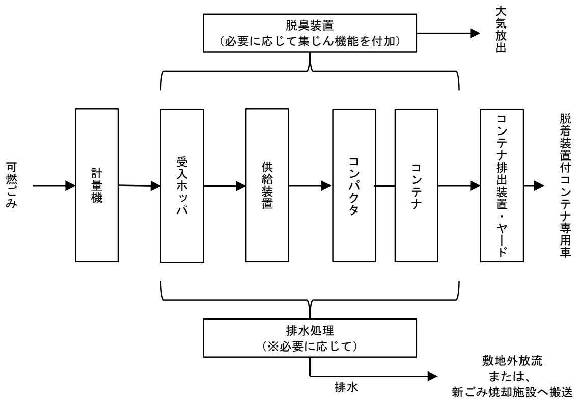
図 8-1 コンパクタ方式の基本処理フロー
