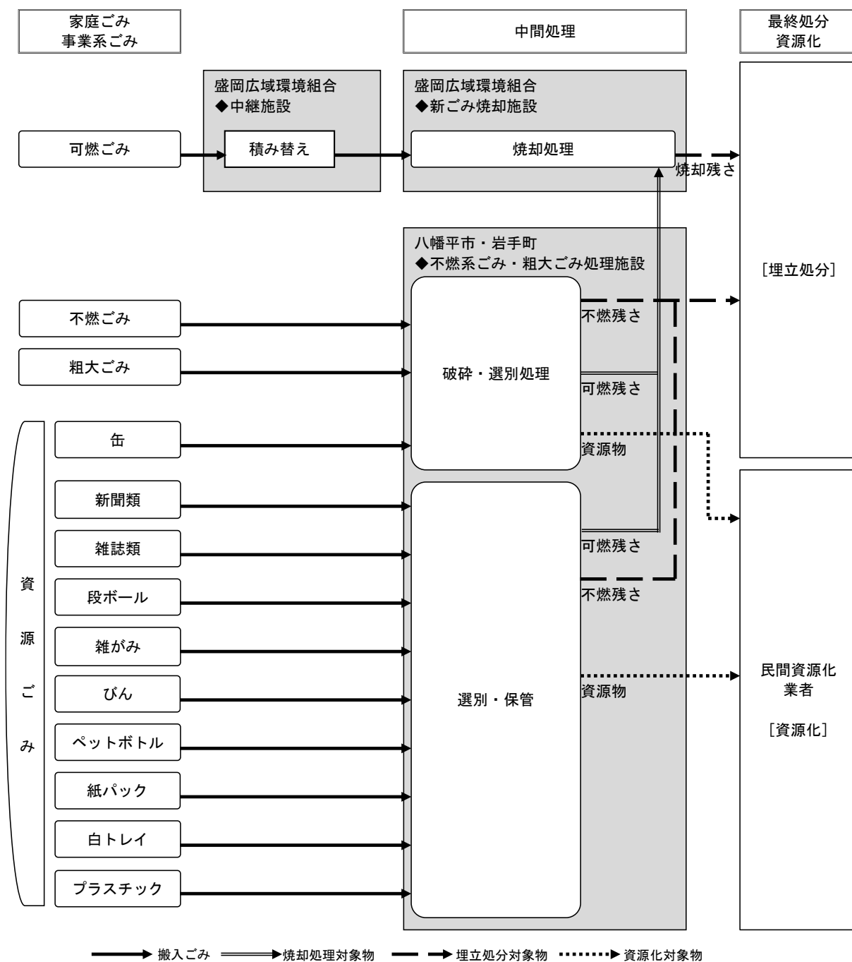
図 5-6 中継施設稼働後のごみ処理体系（岩手町）
